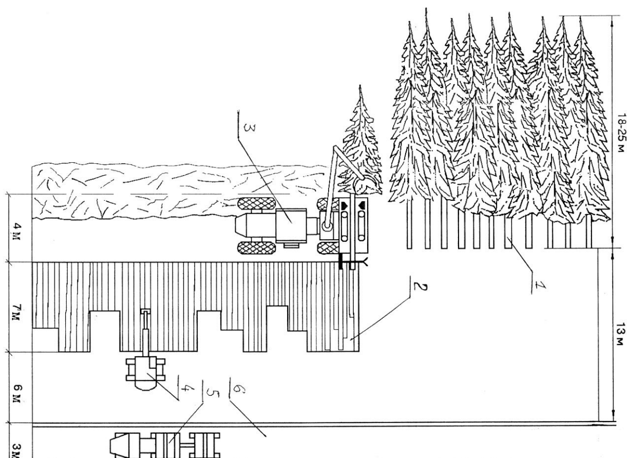
Рис.2.6.8 Схема верхнего склада при машинной выработке сортиментов.
