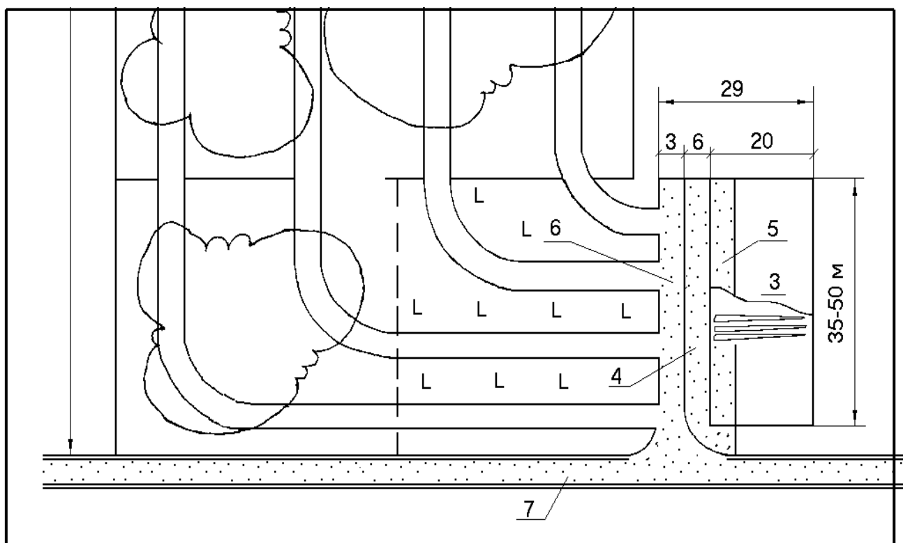
Рис. 2.6.4 Схема погрузочного пункта при трелевке хлыстов за вершину с тупиковым заездом лесовозов под погрузку.
