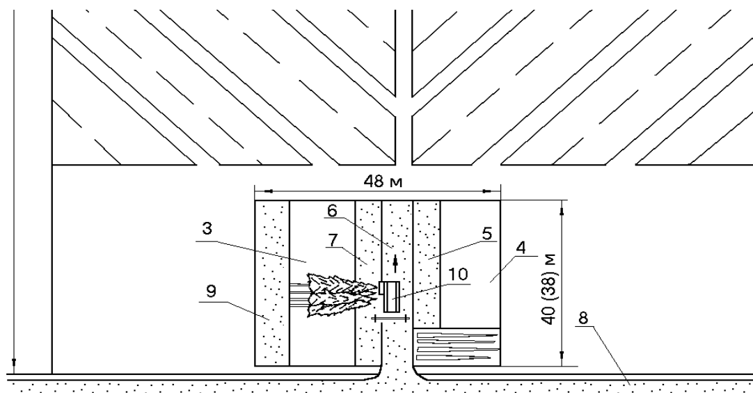
Рис.2.6.6. Схема верхнего склада при трелевке деревьев за комли с тупиковым заездом лесовозов под погрузку
