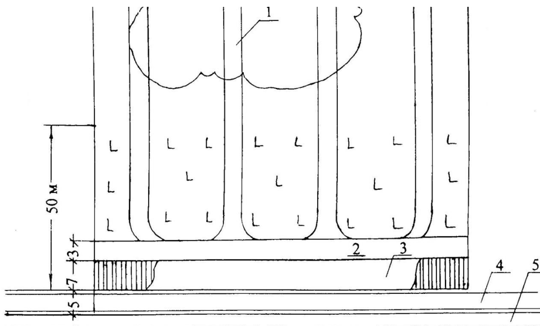
Рис. 2.6.7. Схема верхнего склада при трелевке сортиментов форвардером.
