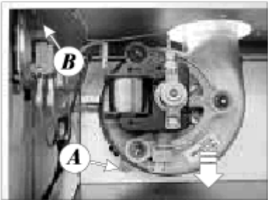
Рис. 19 – Монтаж вентилятора
